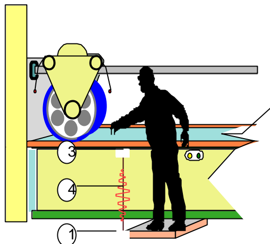
fig.2 - dispositivo di blocco macchina con sistema capacitivo
