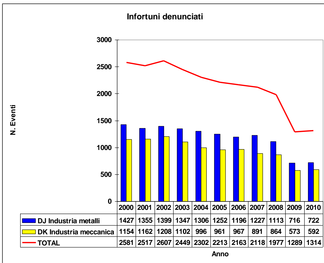
Grafico 9: Infortuni denunciati (2000-2010) settore metalmeccanico
