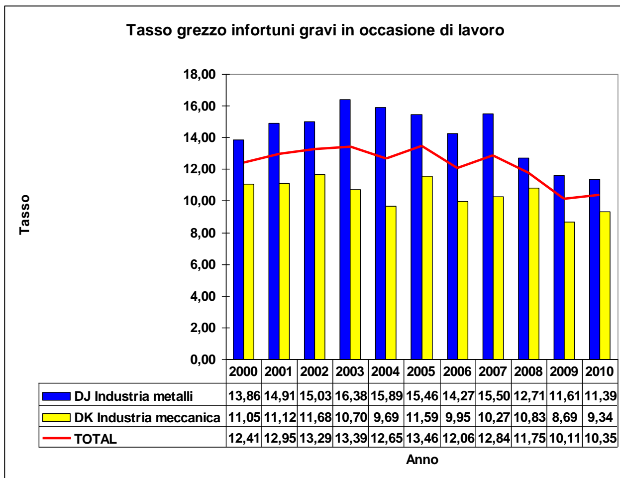
Grafico 14: Indice di incidenza (Tasso grezzo) degli infortuni “gravi” in occasione di lavoro del settore metalmeccanico: andamento 2000- 2010
